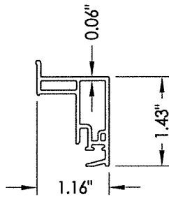
4 LOCK STILE
